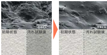
【従来床】
